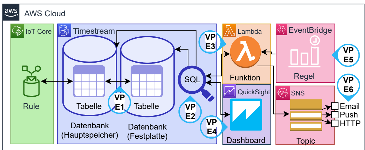
Abb. 43: Bausteinsicht
